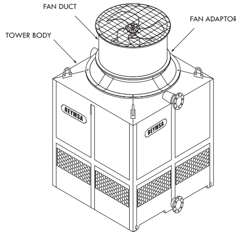
Figure A-35: Fan adaptor in single fan tower
